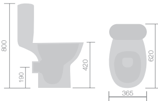
W365 H800 D620 £305
